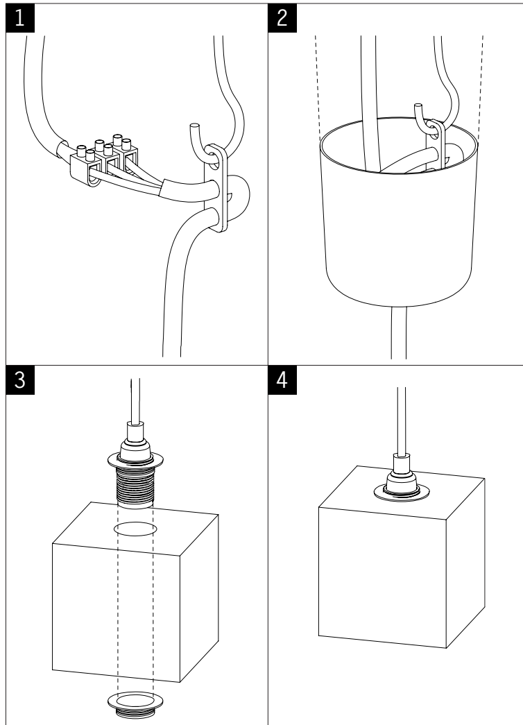
B6 Beton Hängeleuchte / B6 Concrete pendant light
