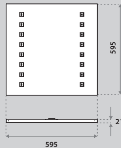
Aviora FL 2L 595x595 (IP20)
