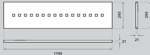
Aviora FL 2L 1195x295 (IP20)
