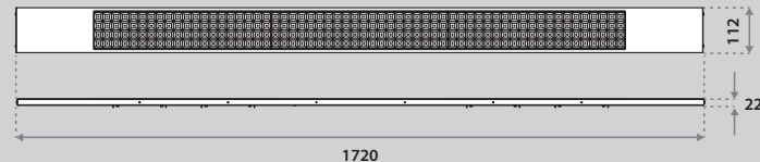
Linessa 3L 1720x112 (IP20)
